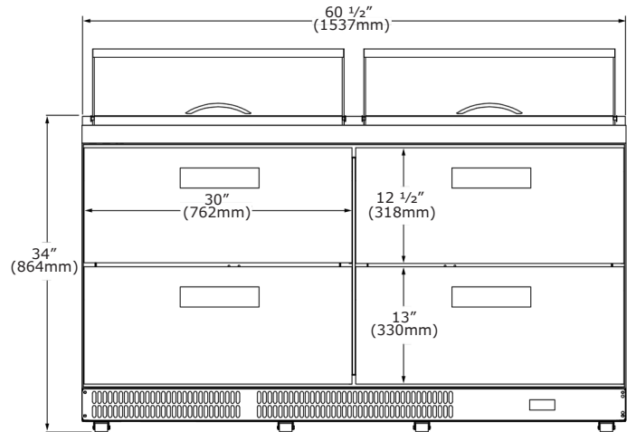
Front (UCMT160-SS91A)
