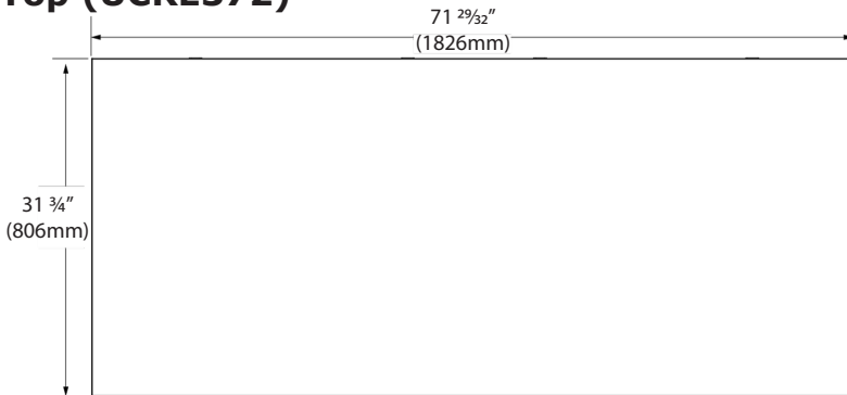
Top (UCRE372)
